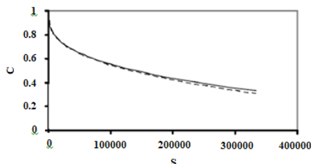
Figura 1: Exemplo de curvas C vs S, considerando ou não o efeito da temperatura medida na superfície dos CPs, adaptado de Lundström e Ekblad (2006)
