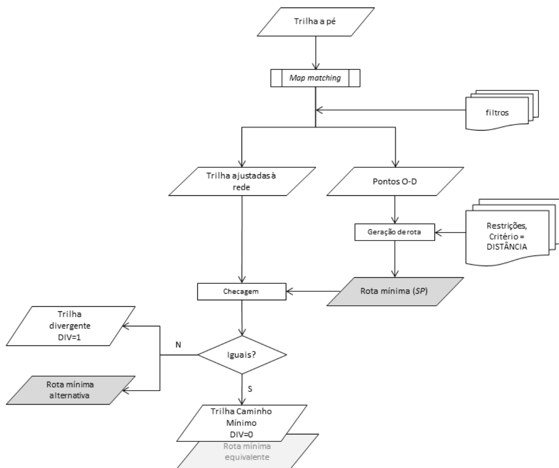
Figura 6: Fluxograma para a geração dos caminhos mínimos e checagem das rotas realizadas.
