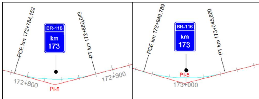
Figura 2 - Exemplo de correção do erro do SNV em relação ao marco quilométrico
