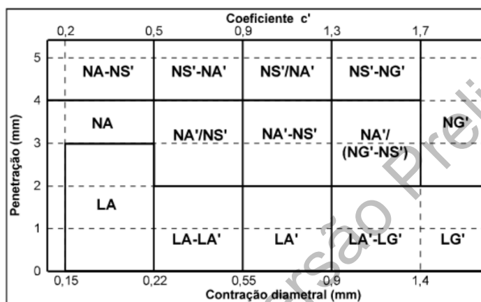
Figura 2: Carta de Classificação do Método das pastilhas.
