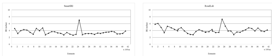
Figura 5: Gráfico de linhas (SmartIRI e RoadLab)
