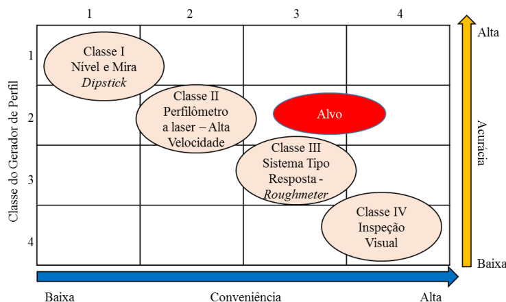
Figura 3: Classificação dos smartphones em relação aos equipamentos de medição de irregularidade (Tomiyama et al. , 2012)
