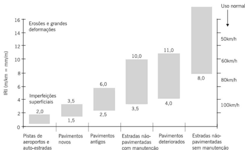
Figura 2: Diversas faixas de variação do IRI (Karamihas e Sayers, 1998)
