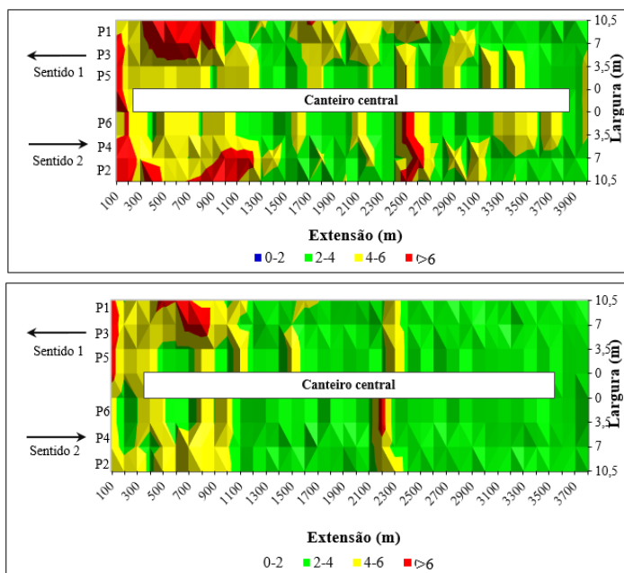
Figura 7: Gráfico tridimensional – RoadLab (acima) e SmartIRI (abaixo)
