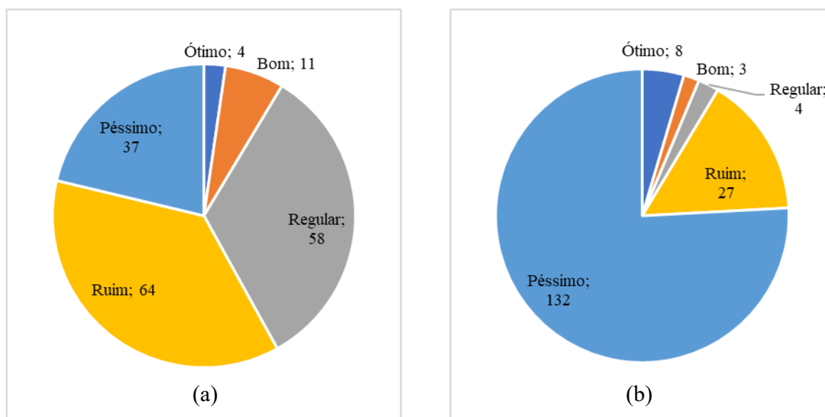
Figura 1: Condições dos segmentos obtidos do IGG (a) e do IGG_{TS} (b).
