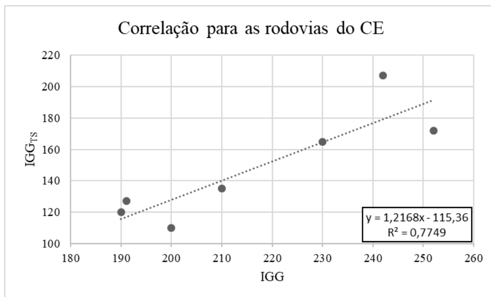
Figura 3: Gráfico de correlação obtido entre IGG e IGG TS para a BR-230/CE
