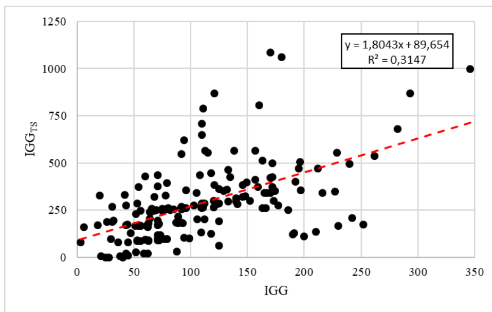
Figura 2: Gráfico de correlação obtido entre o IGG e o IGG_{TS} .
