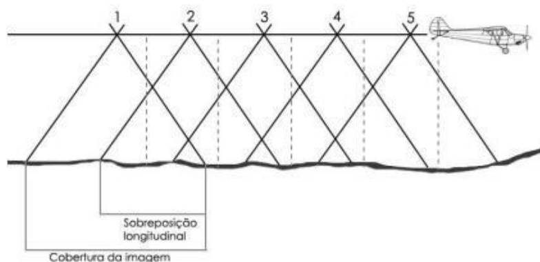
Figura 1: Exemplificação de levantamento aéreo com sobreposição longitudinal
