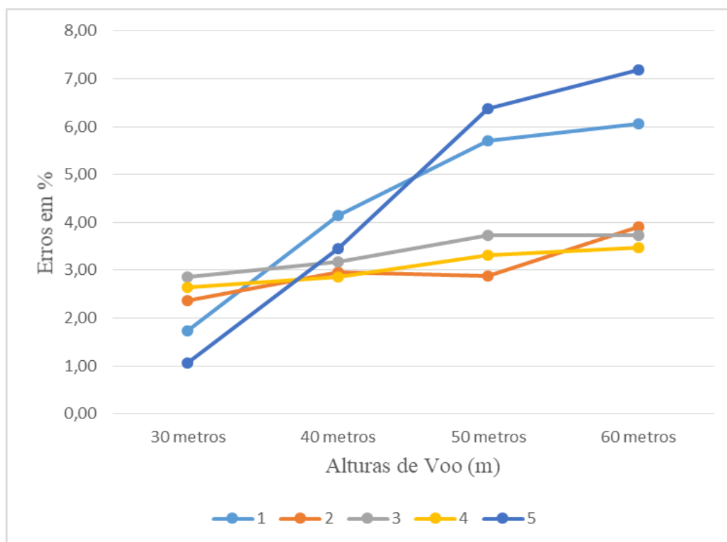
Figura 7: Comparação dos erros percentuais entre cada defeito levantado.
