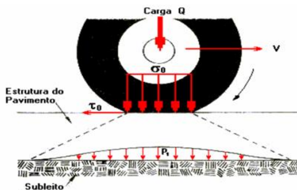
Figura 1: Cargas no Pavimento (Santana, 1993)
