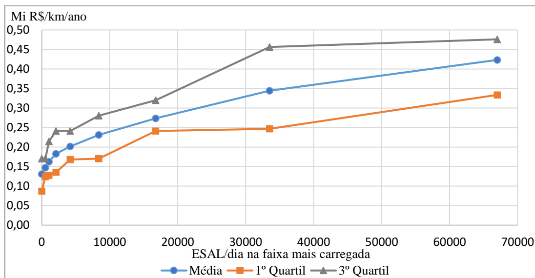
Figura 2: Custos de manutenção versus ESAL por dia na faixa mais carregada
