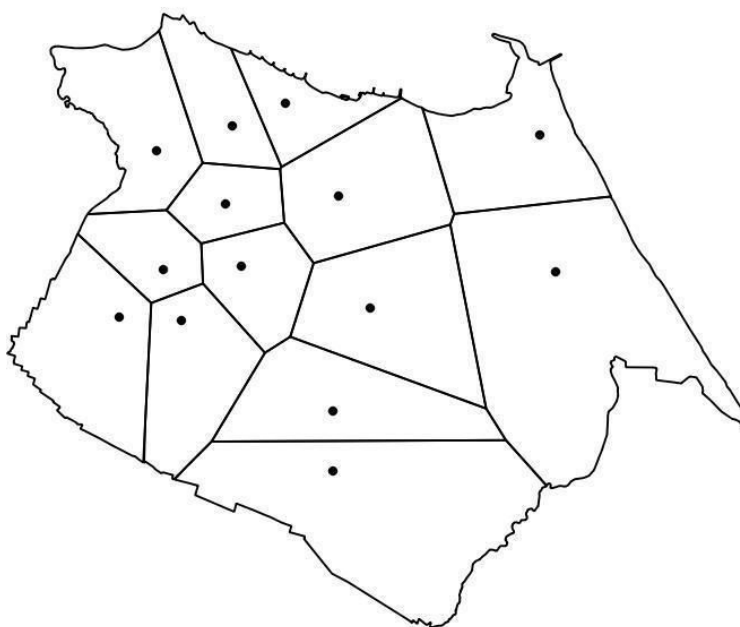
Figura 2: Polígono de Thiessen das estações pluviométricas
