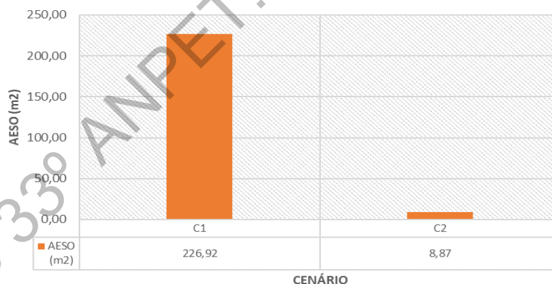
Figura 6: Área Equivalente de Suscetibilidade Operacional do segmento R20C1
