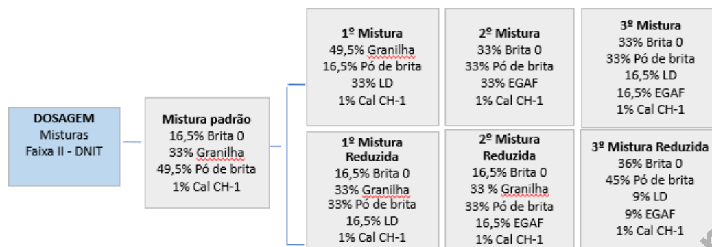
Figura 2: Dosagem das misturas - Faixa II DNIT
