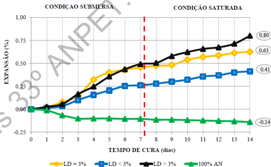
Figura 6: PTM Modificado
